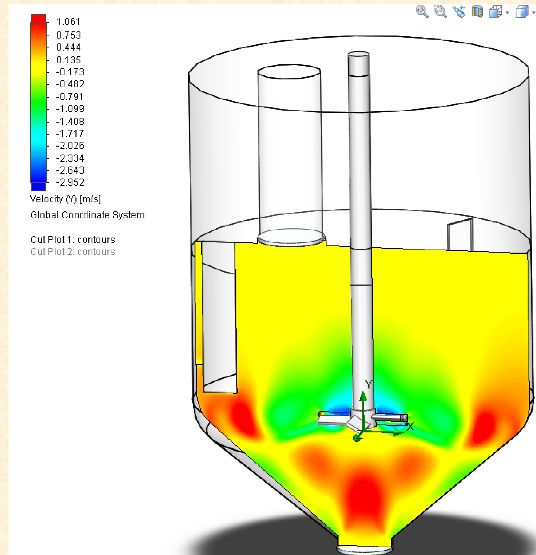
Профиль скоростей в продольном разрезе реактора
