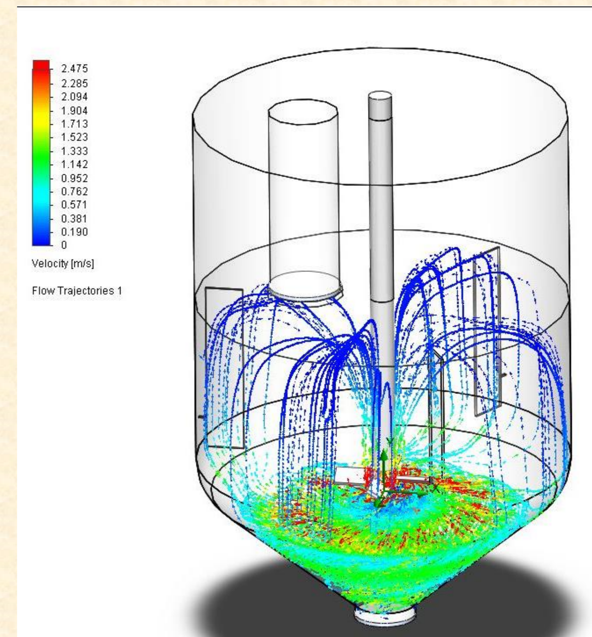
Линии тока жидкости в объеме реактора
